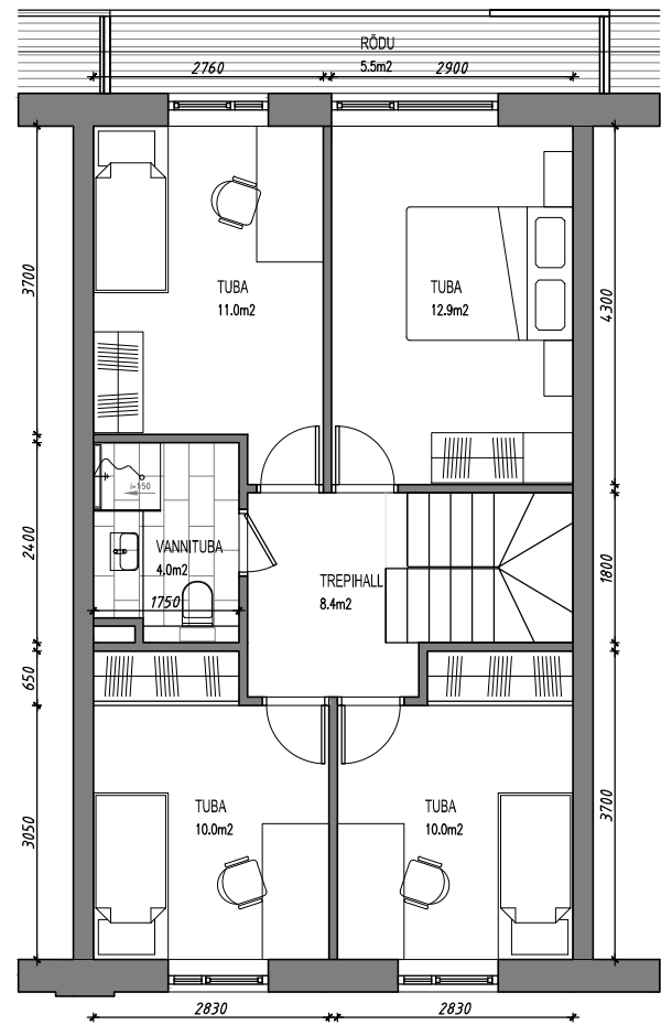
TEINE KORRUS, 5-TOALINE
